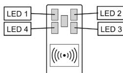
Figure 92 - Disposition des LED sur les lecteurs
